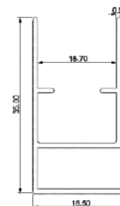
2. Рамный профиль
